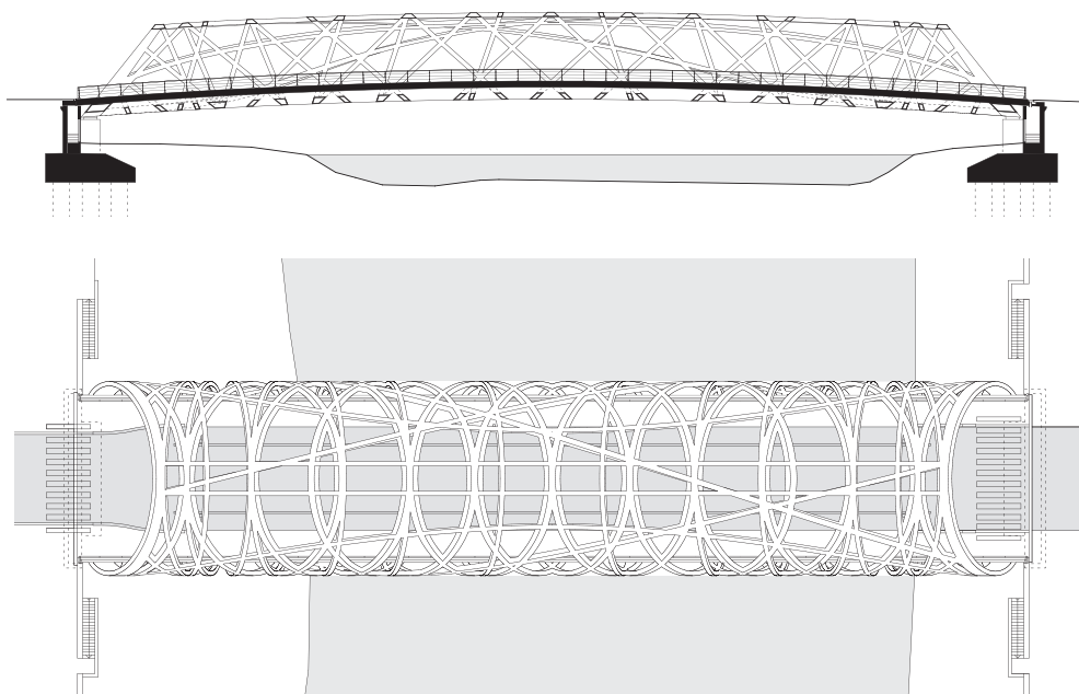
Längsschnitt, Aufsicht, M 1:750
