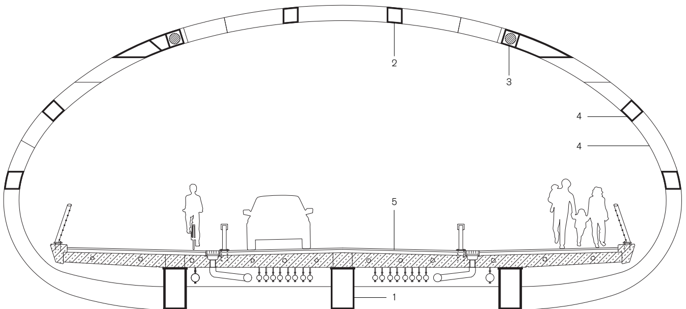
Querschnitt, M 1:100
